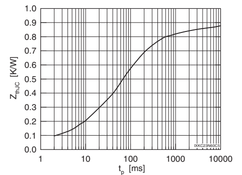
Fig. 12 Max. transient thermal impedance
