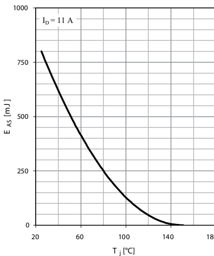
Fig. 10 Avalanche energy
