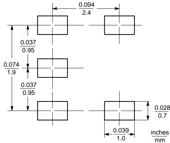
TSOP-5
