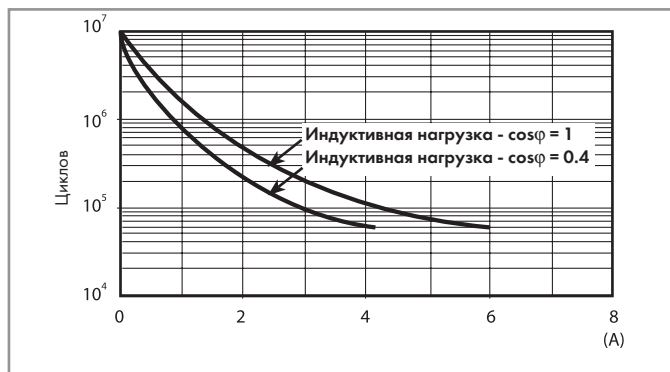
F 34 - Электрическая долговечность (АС) при номинальной нагрузке
