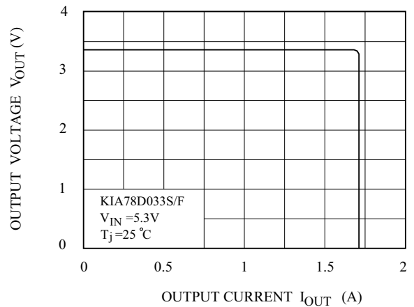
Fig. 9 V_{OUT} - I_{OUT}
