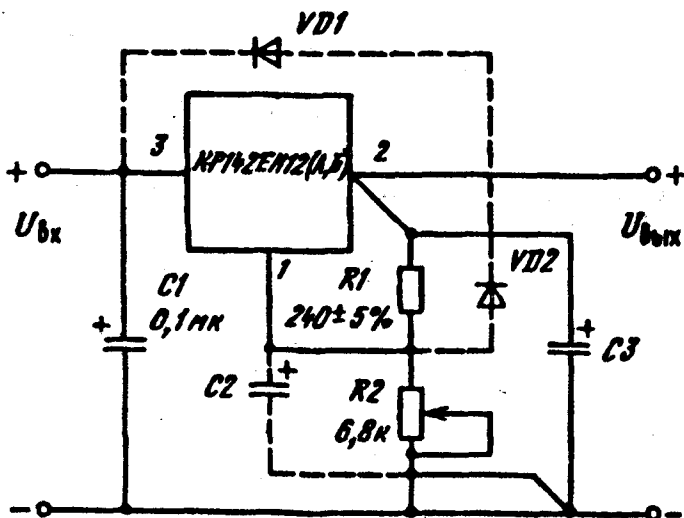
Типовая схема включения КР142ЕН12 (А, Б)
