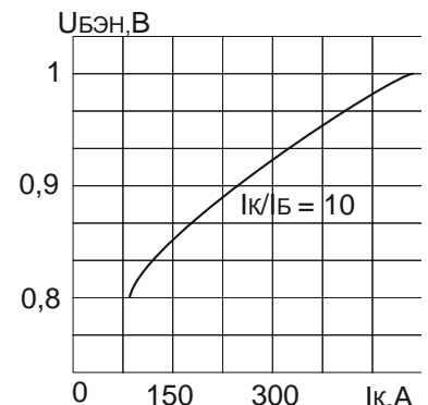
Зависимость напряжения насыщения база-эмиттер от постоянного тока коллектора
