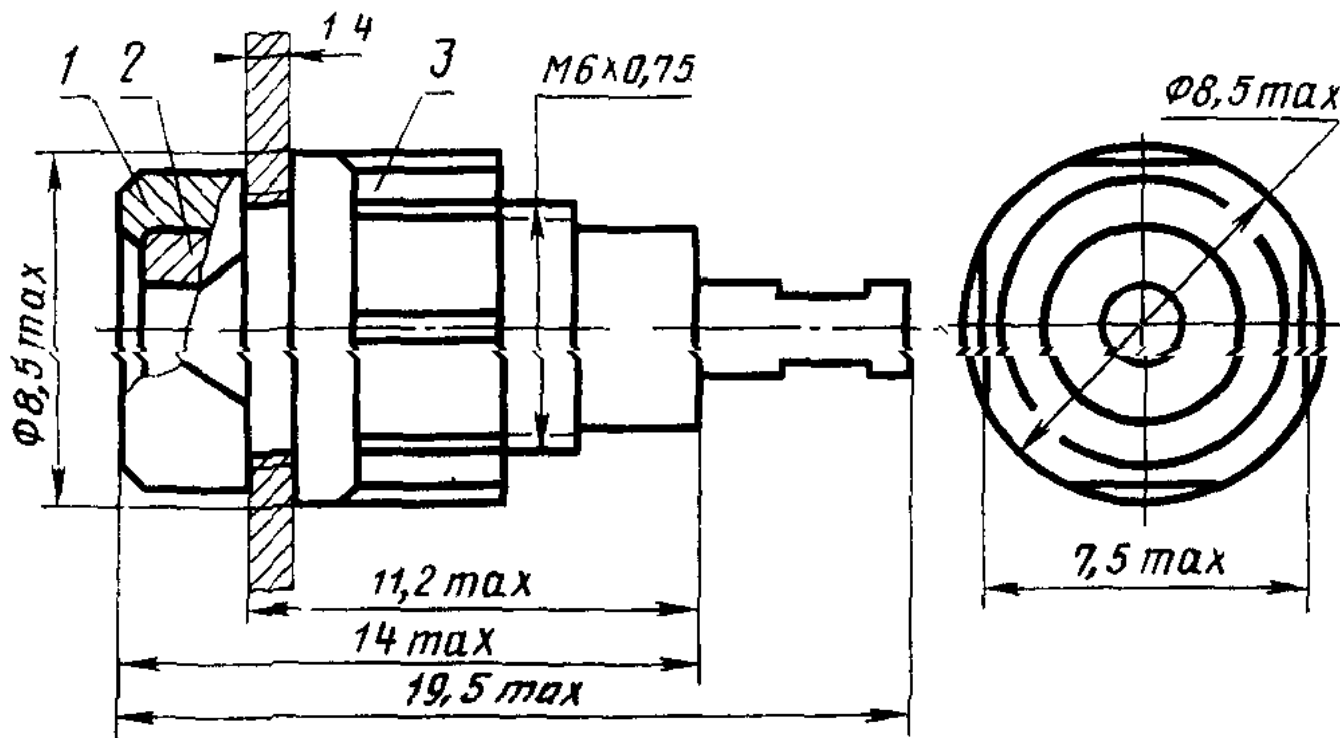
1—корпус; 2—втулка; 3—гайка
