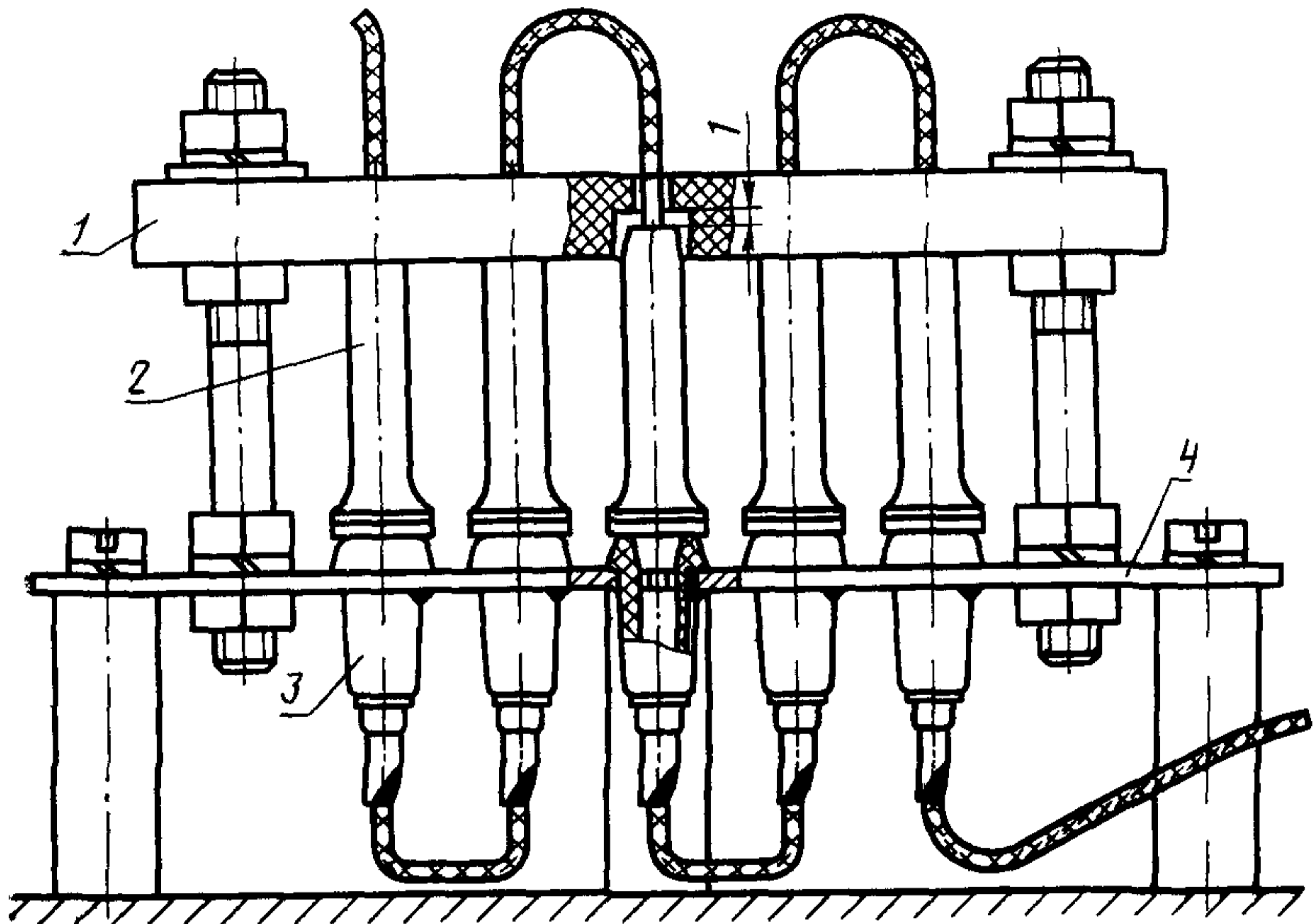
1—планка; 2—штепсель; 3—гнездо; 4—панель
