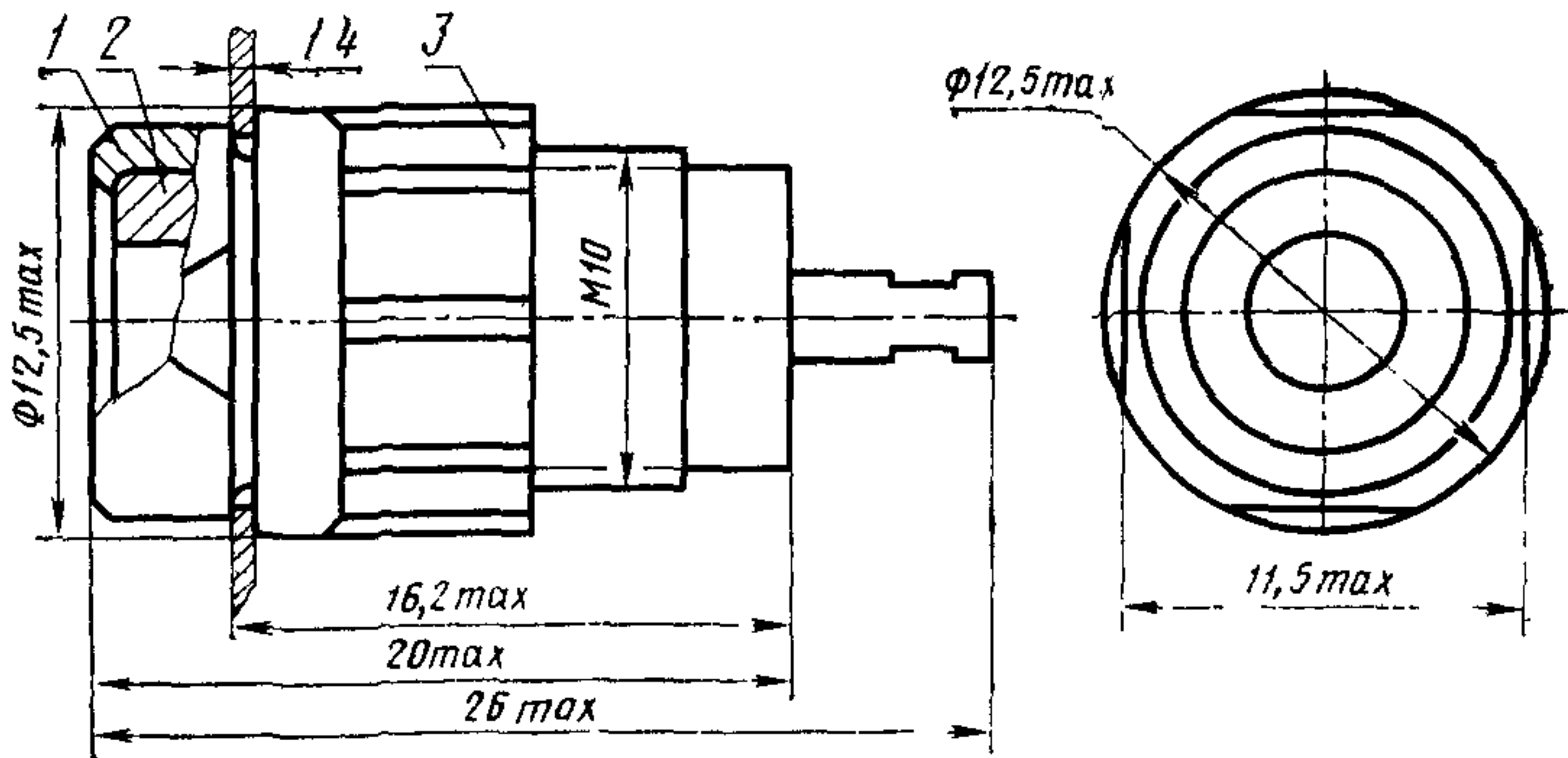
1—корпус; 2—втулка; 3—гайка
