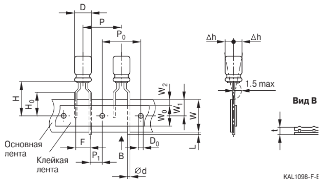
Рис. 1 Упаковка на ленту, диаметр корпуса D < 10 мм
