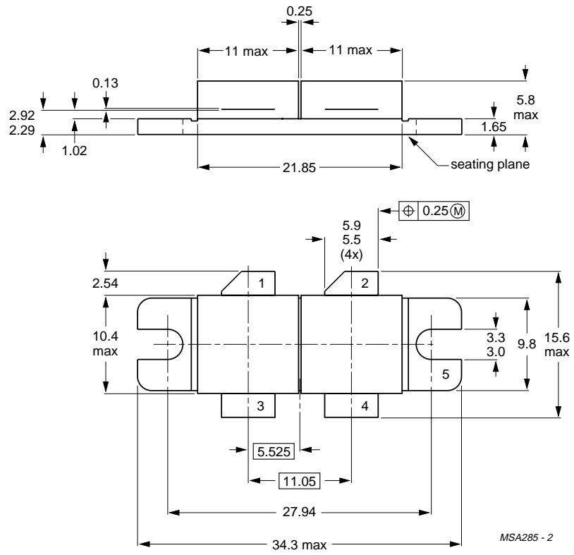
Fig.27 SOT262A1.
