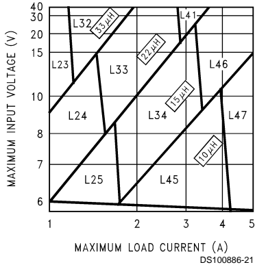
FIGURE 3. LM2678-3.3
