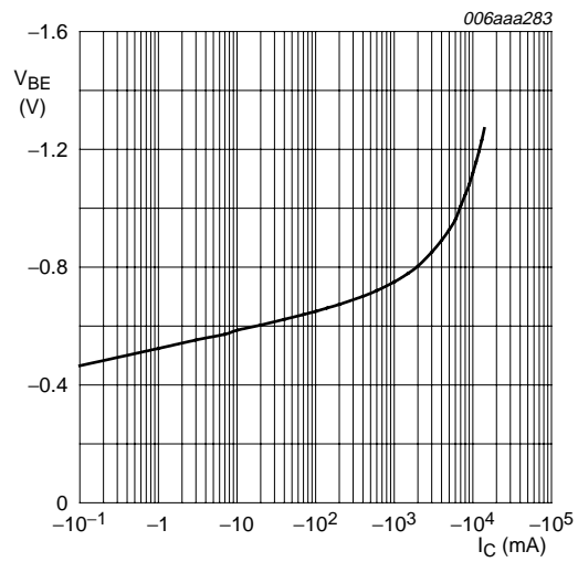
V_{CE} = -2\text{ V} (1) T_{amb} = 25\text{ °C}
