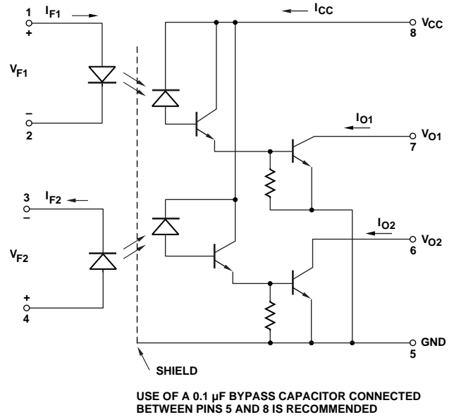
HCPL-273L/HCPL-073L
