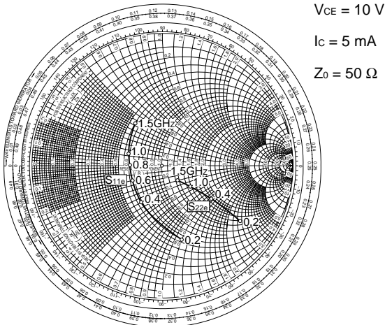
S-PARAMETER
