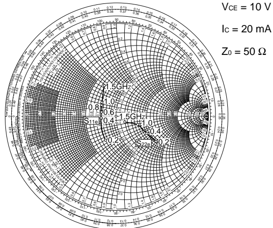
S-PARAMETER
